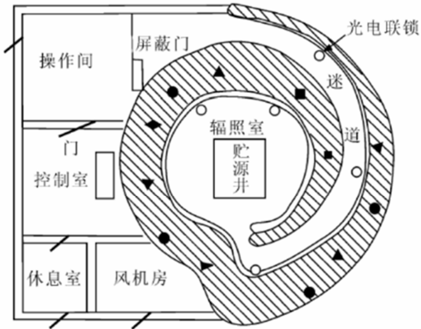
图 1 ^{60}\text{Co} 辐照站平面示意图
