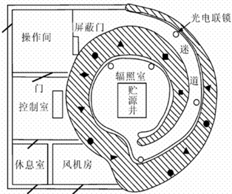
图 1 ^{60}\text{Co} 辐照站平面示意图
